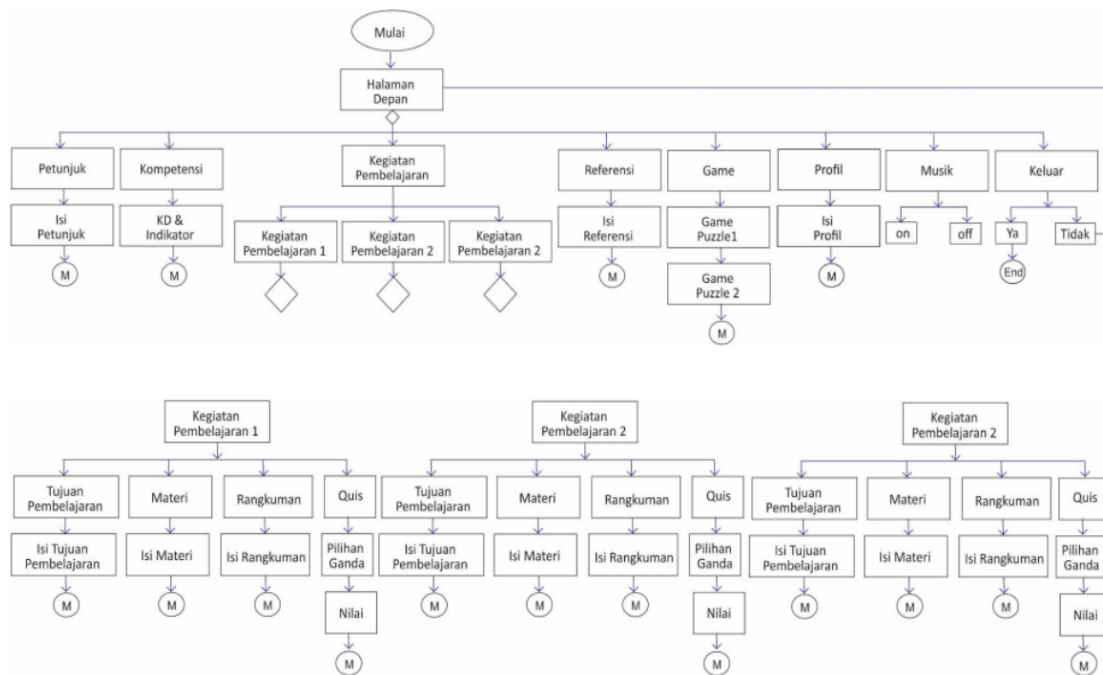
Gambar 2: Flowchart Multimedia Pembelajaran Interaktif
